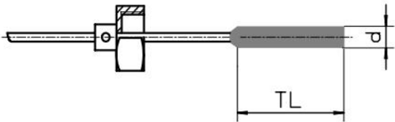
Fühler F4-1: lose Überwurfmutter auf Fernleitung verschiebbar
