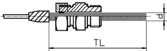
Fühler F7: glatter Fühler (F1) mit Klemmringverschraubung
