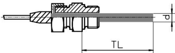
Fühler F6: lose Überwurfmutter (F4) mit Anschlussverschraubung
