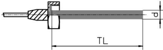
Fühler F4: lose Überwurfmutter
